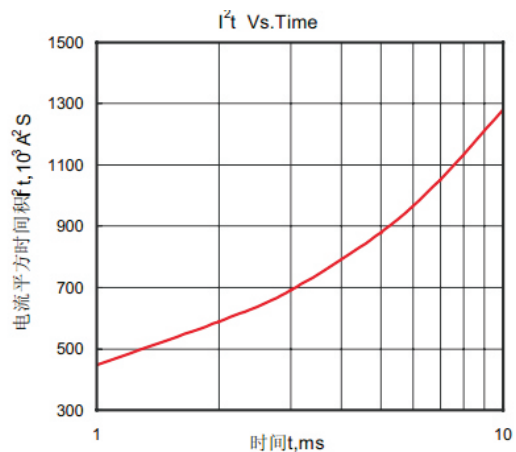
Fig.8 I^2t 特性曲线
