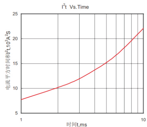
Fig.6 I^2t 特性曲线
