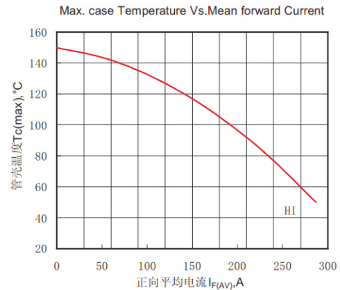
Fig.4 管壳温度与平均电流的关系曲线
