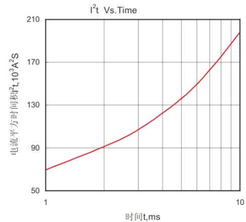
Fig.4 I^2t 特性曲线
